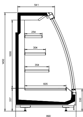
NordicStar SV5 30-89-145
