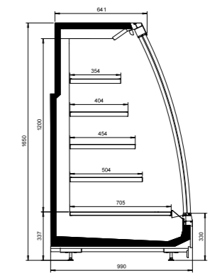
NordicStar SV5 30-99-165
