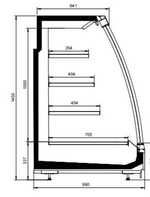
NordicStar SV5 30-99-145
