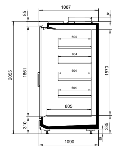
NordiLine MD5 30-109-206 GD
