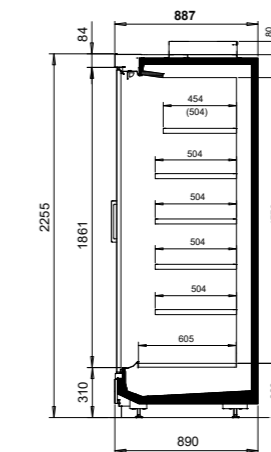
NordiLine MD5 30-89-226 GD
