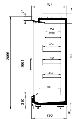
NordiLine MD5 30-79-206 GD*
