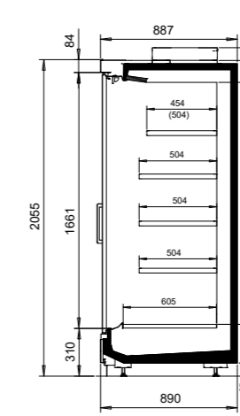
NordiLine MD5 30-89-206 GD
