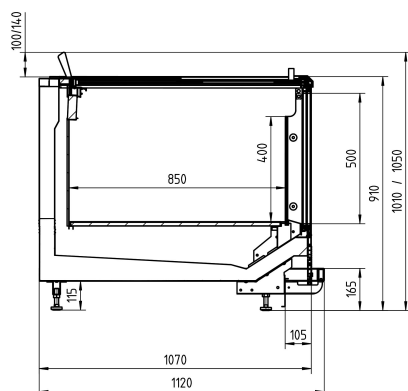
IS7-200 - EOL
